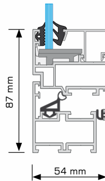
ablakmetszet
