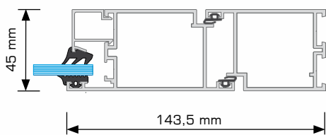
ajtómetszet
